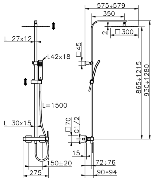
QT 0R4032 CombiDoccia Monocomando CombiShower Mixer CombiDouche Mitigeur
