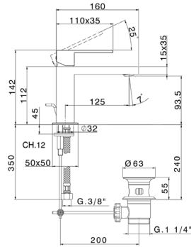
NE 000514 Monocomando Lavabo Basin Mixer Mitigeur Lavabo
