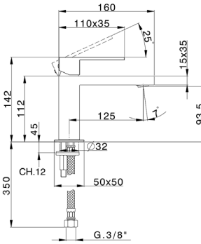
NE 000544 Monocomando Lavabo Basin Mixer Mitigeur Lavabo
