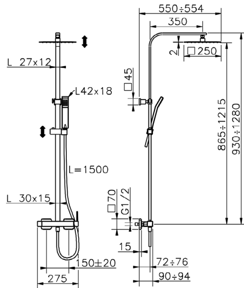
QT 0R4031 CombiDoccia Monocomando CombiShower Mixer CombiDouche Mitigeur
