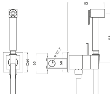
EG 007945 Set Miscelatore Doccetta Igienica Bidet Hand Shower Mixer Set Kit Mitigeur Douche d'Hygiène
