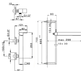
NE 000464 Completo Monocomando Doccia Shower Mixer Set Ensemble Mitigeur Douche
